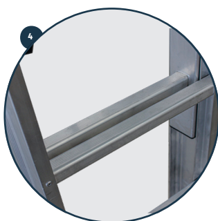
4 Peldaños engastados y remachados Rungs set and riveted Échelons sertis et rivetés Degraus inseridos e rebitados
